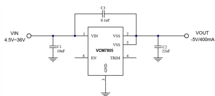
负压输出
