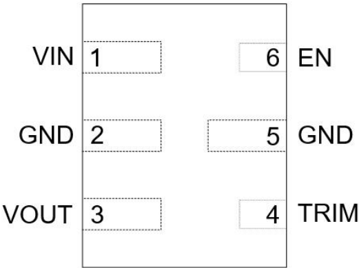
降压输出
