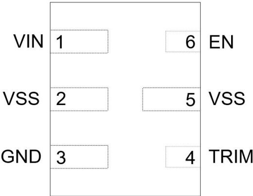
负压输出
