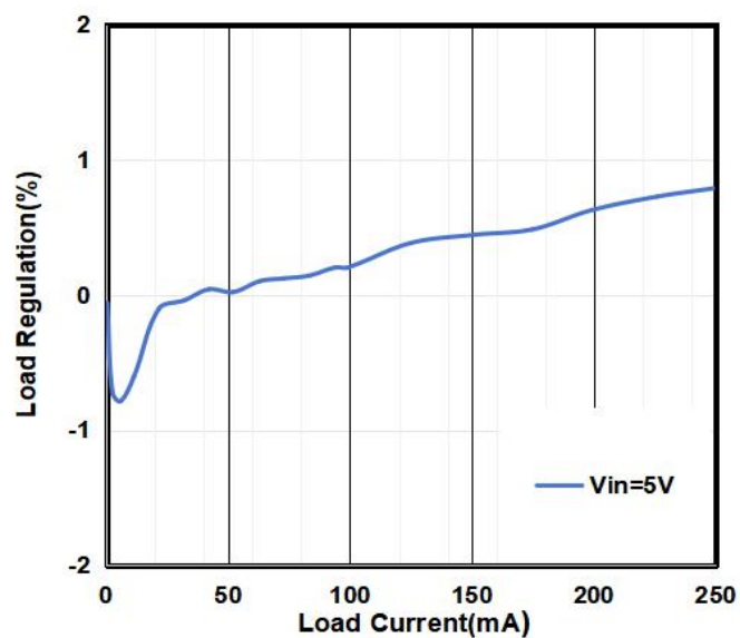
负载调整率
