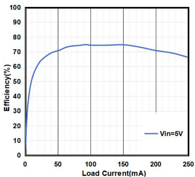
效率曲线
