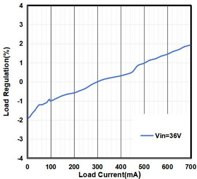
负载调整率
