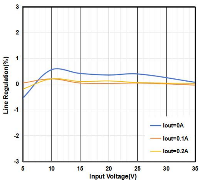
电源调整率
