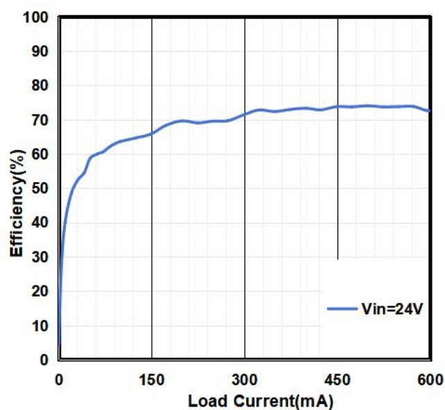
效率曲线
