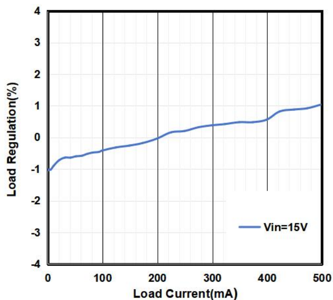
负载调整率
