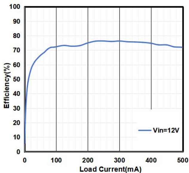
效率曲线
