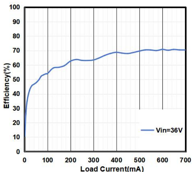
效率曲线
