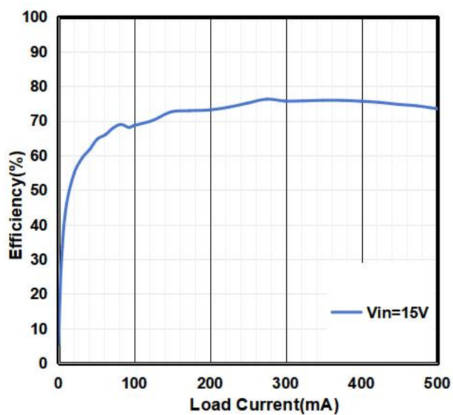
效率曲线
