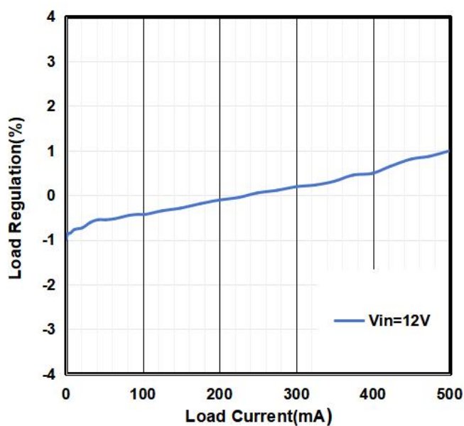
负载调整率
