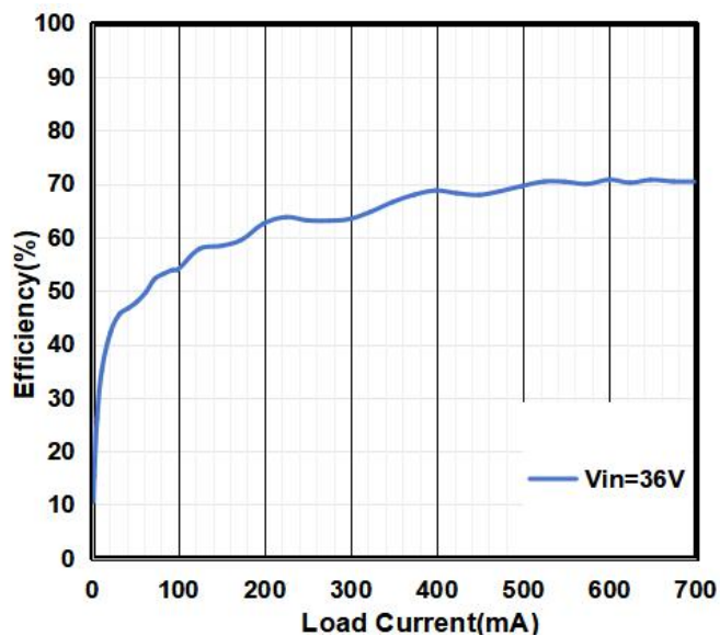
效率曲线
