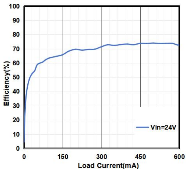
效率曲线
