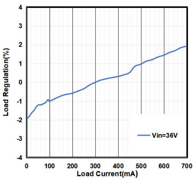
负载调整率
