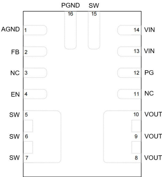
LGA-16 (3.5mmx2.5mmx1.2mm)
