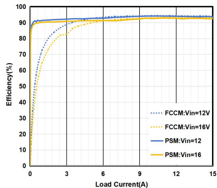
效率曲线 V OUT =5V
