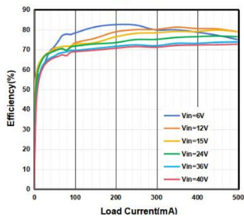
效率曲线
