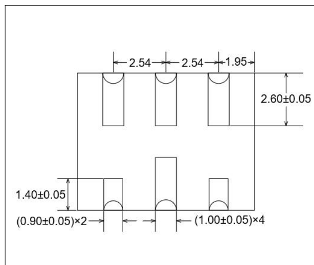
底视图
