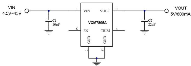
降压输出
