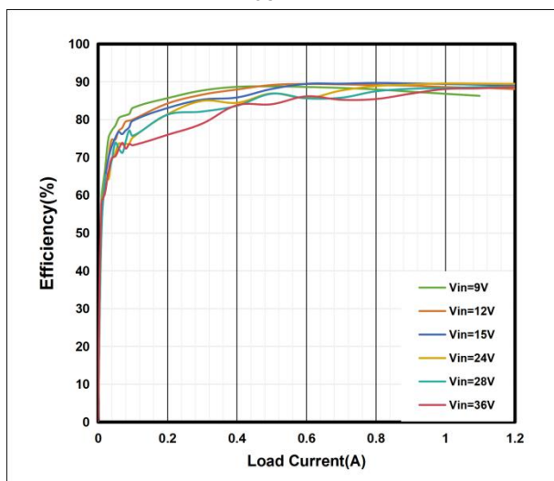
效率曲线
