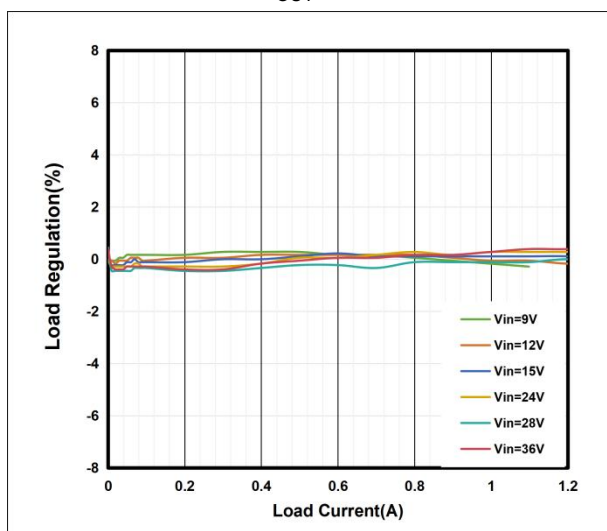
负载调整率
