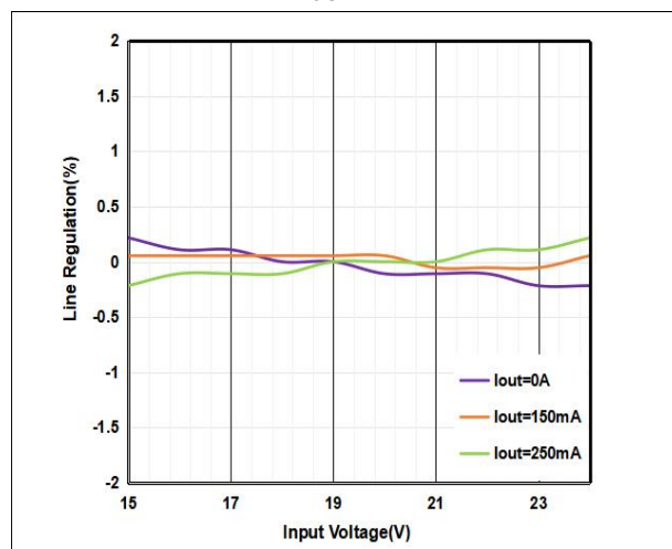
电源调整率
