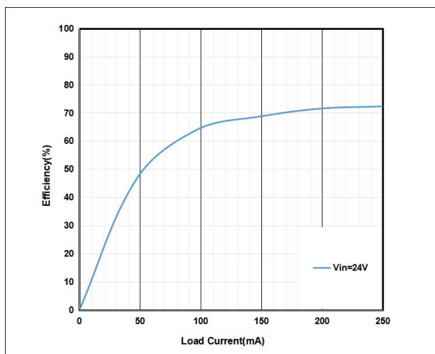
效率曲线
