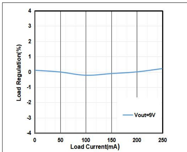
负载调整率
