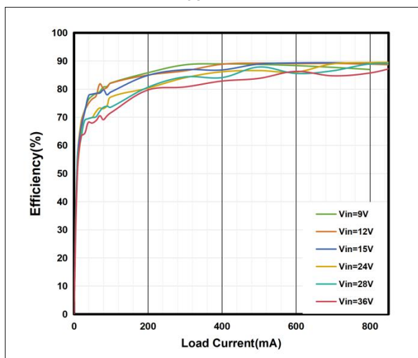
效率曲线
