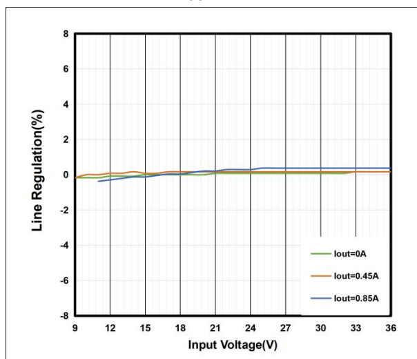
电源调整率
