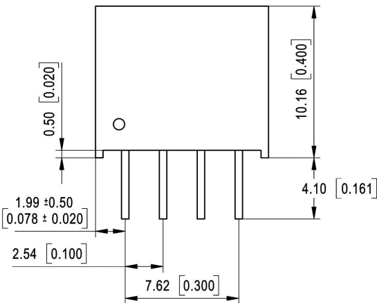
前视图
