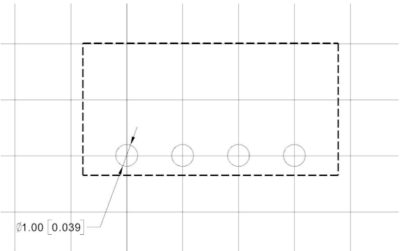
俯视图
