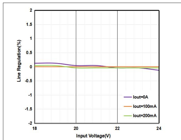
电源调整率
