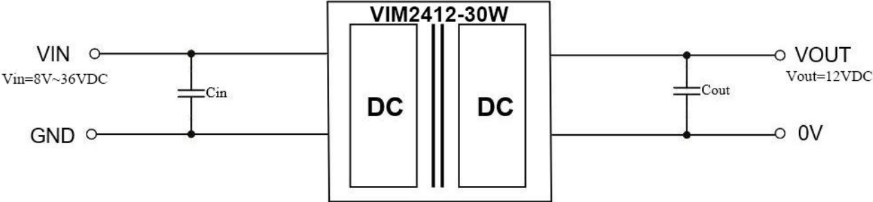
图 1. 典型应用线路图
