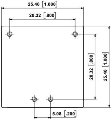
俯视图
