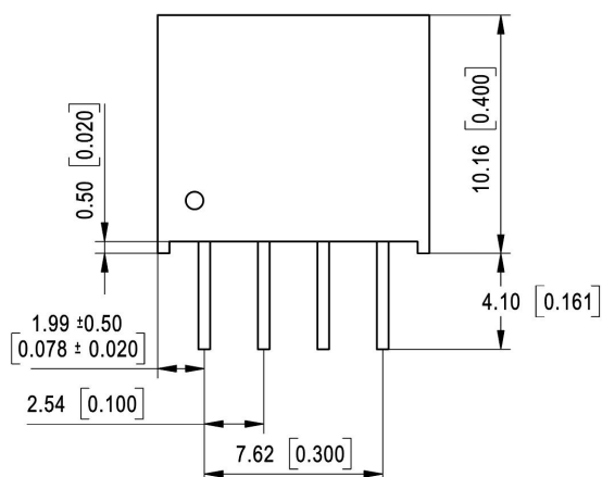
前视图
