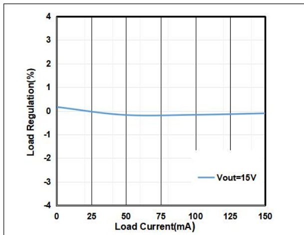
负载调整率
