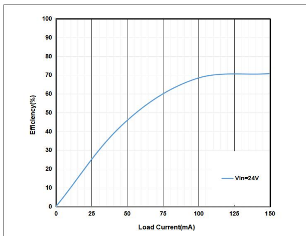
效率曲线
