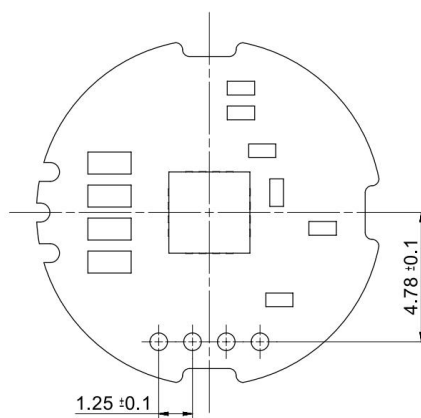
底视图
